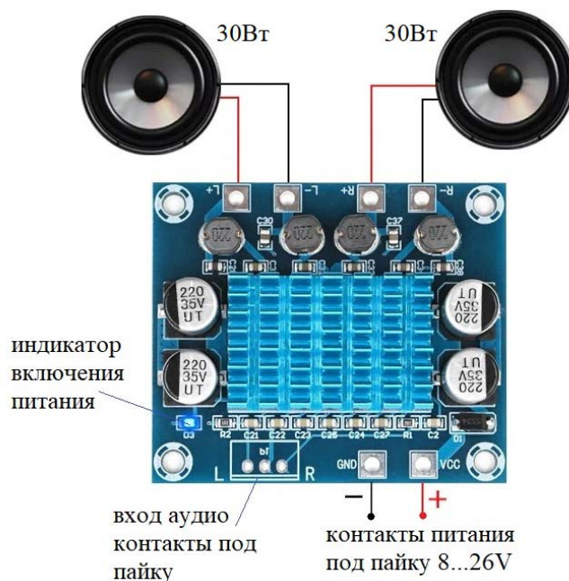
Эскиз подключения
